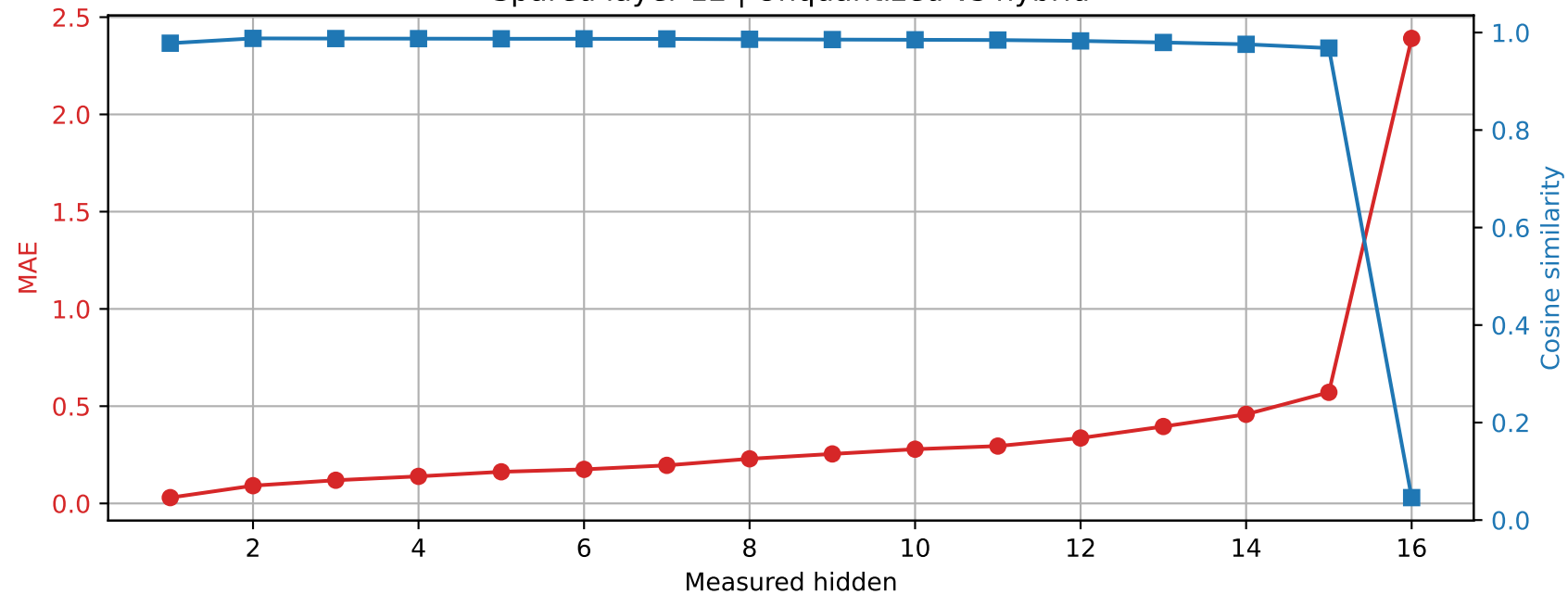
Llama-3.2-1B | Prompt 3 Spared layer 12 | Unquantized vs hybrid
