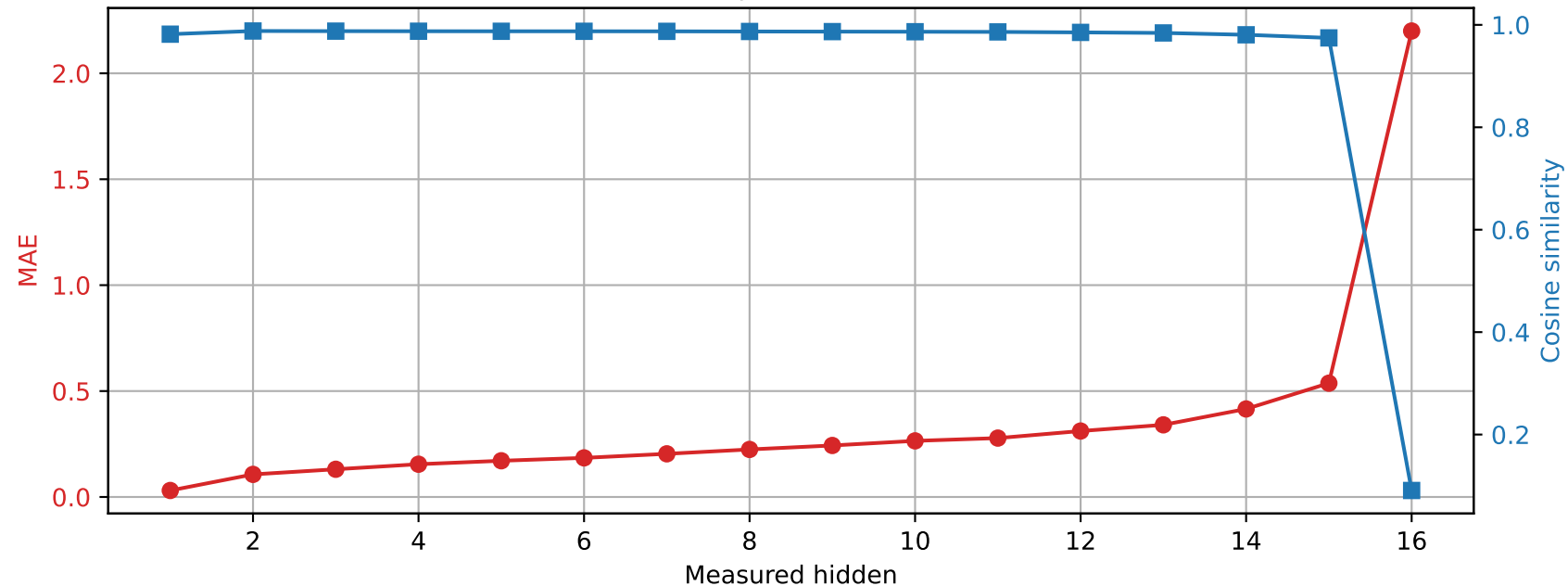
Llama-3.2-1B | Prompt 4 Spared layer 13 | Unquantized vs hybrid
