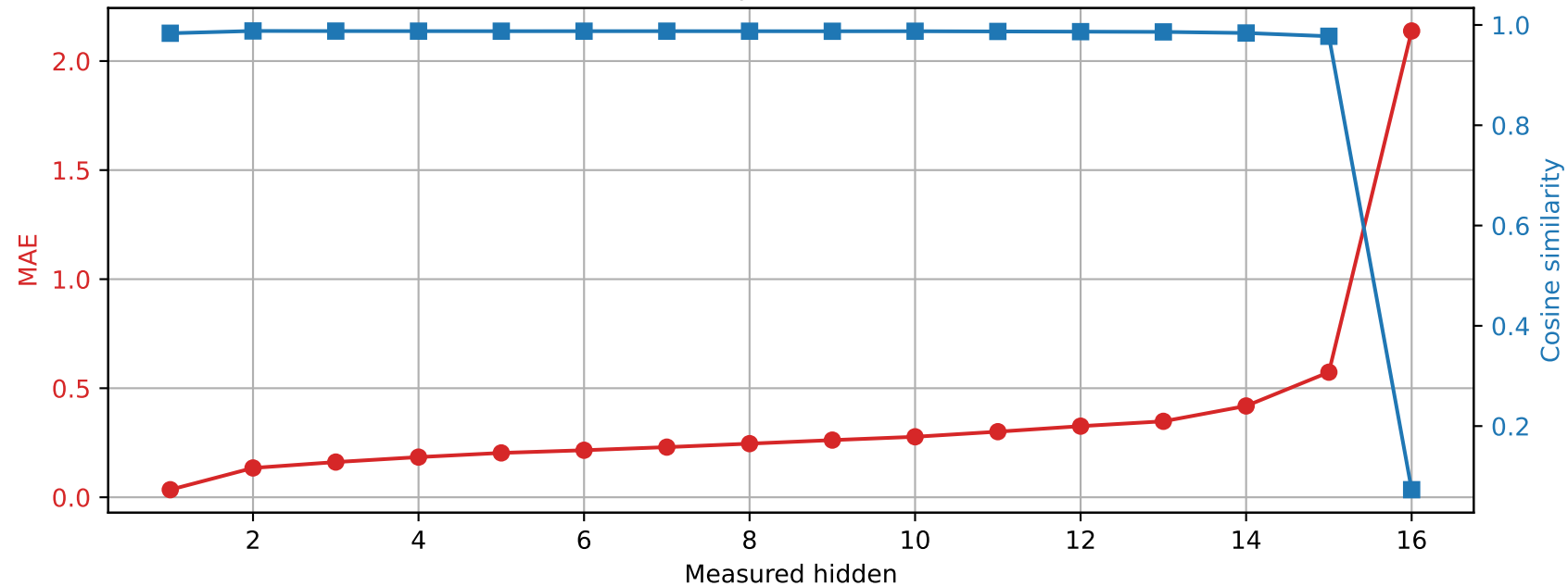
Llama-3.2-1B | Prompt 0 Spared layer 10 | Unquantized vs hybrid
