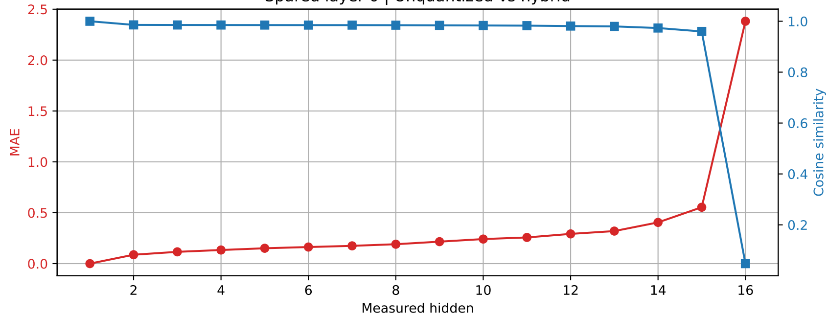
Llama-3.2-1B | Prompt 1 Spared layer 0 | Unquantized vs hybrid
