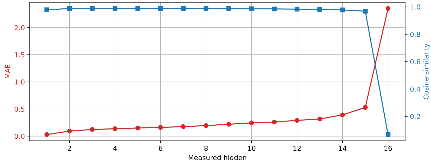
Llama-3.2-1B | Prompt 1 Spared layer 3 | Unquantized vs hybrid
