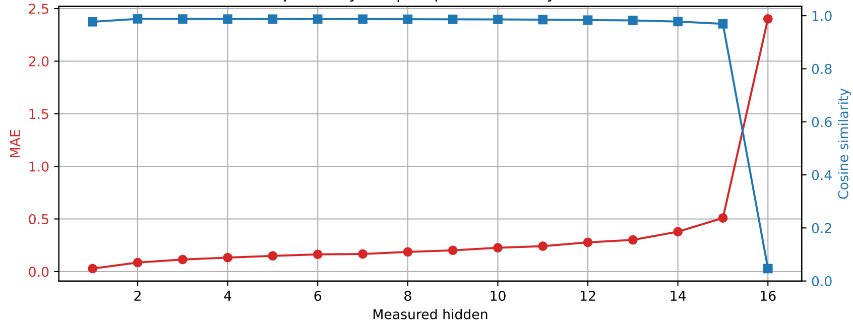
Llama-3.2-1B | Prompt 2 Spared layer 6 | Unquantized vs hybrid
