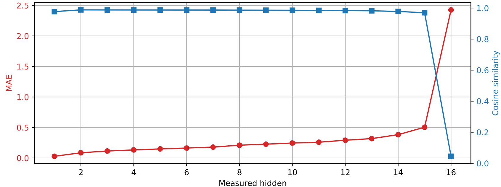
Llama-3.2-1B | Prompt 2 Spared layer 8 | Unquantized vs hybrid
