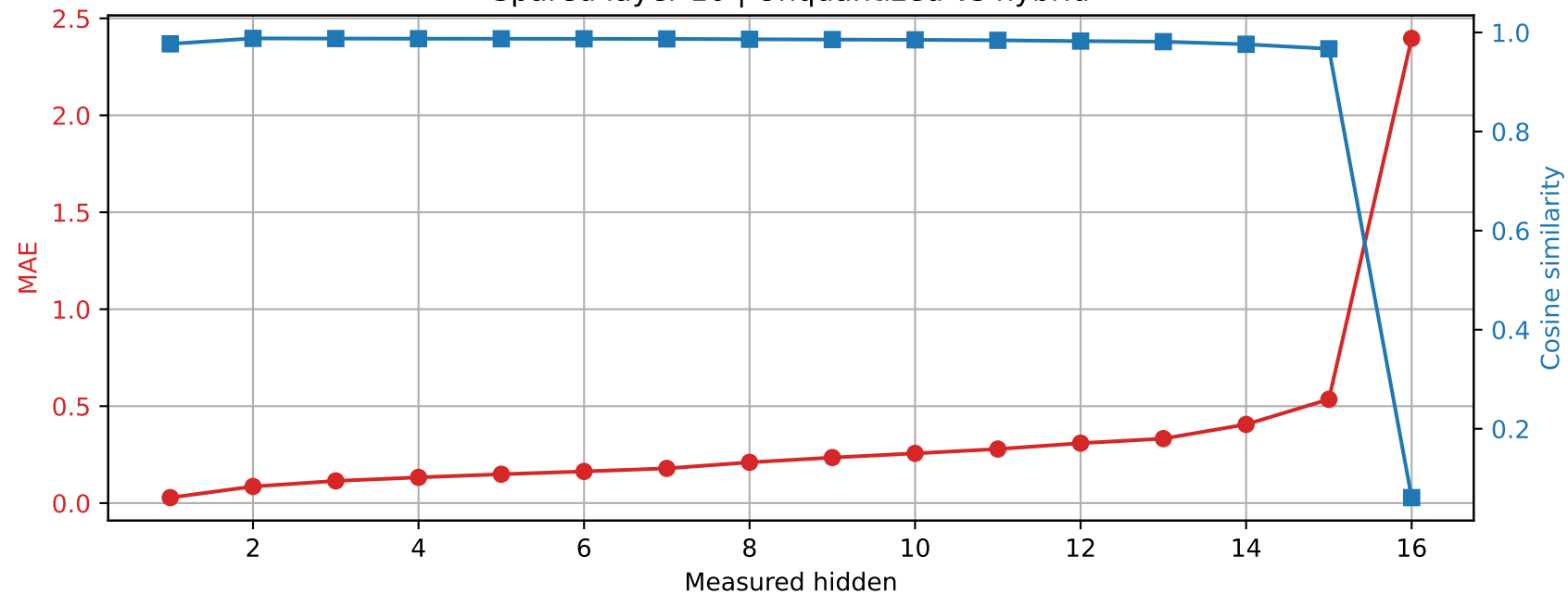
Llama-3.2-1B | Prompt 2 Spared layer 10 | Unquantized vs hybrid
