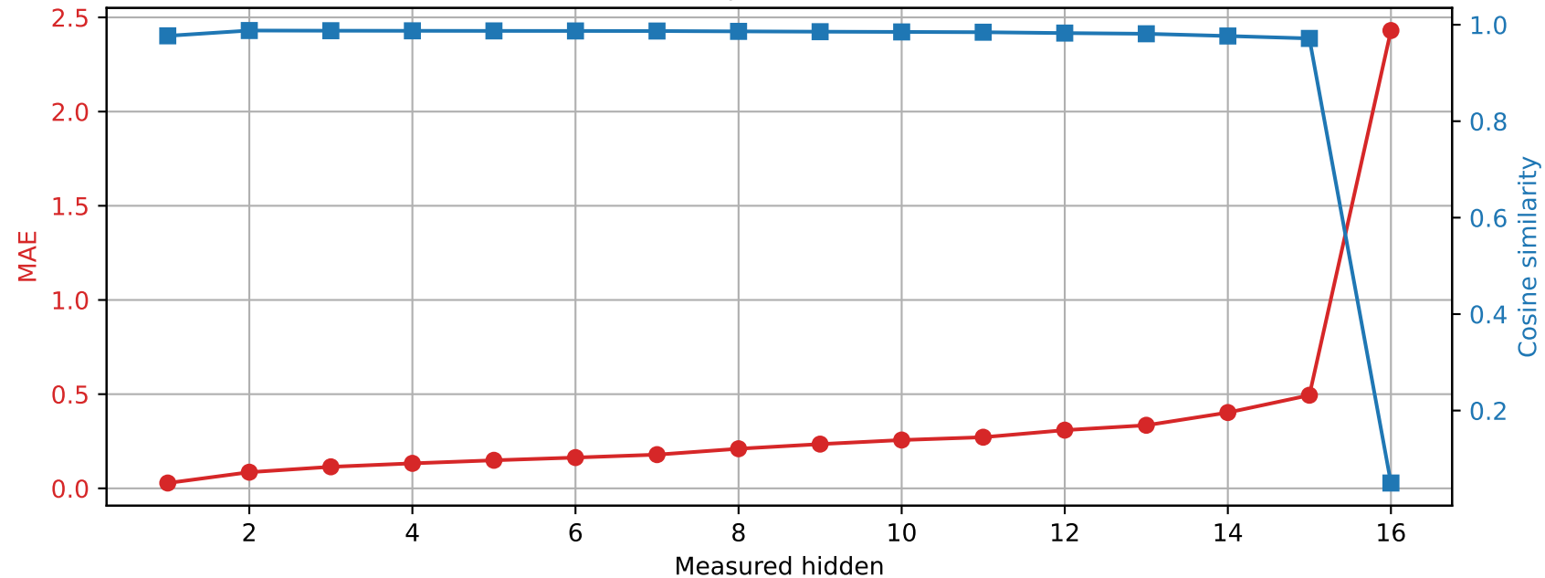
Llama-3.2-1B | Prompt 2 Spared layer 14 | Unquantized vs hybrid
