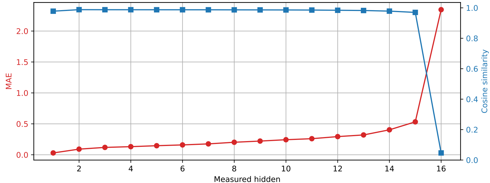
Llama-3.2-1B | Prompt 3 Spared layer 3 | Unquantized vs hybrid
