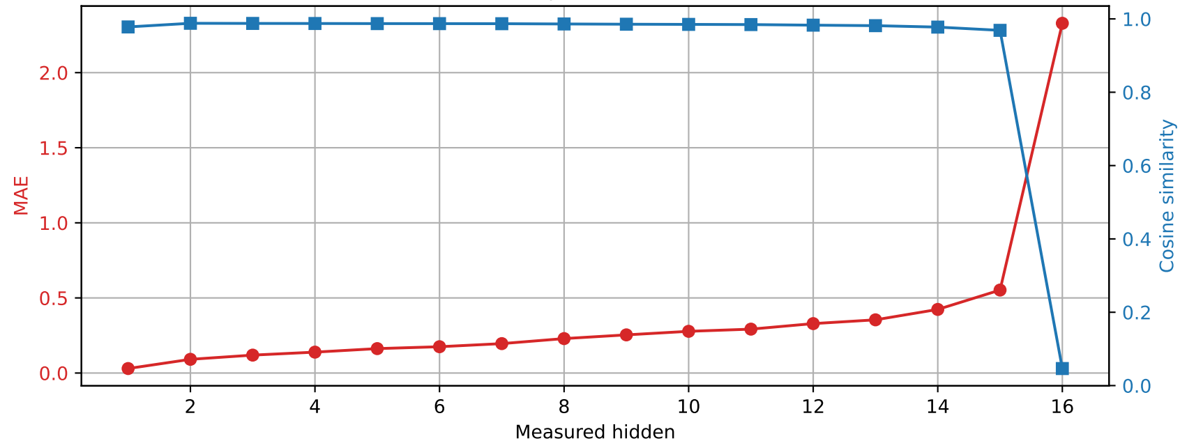
Llama-3.2-1B | Prompt 3 Spared layer 8 | Unquantized vs hybrid
