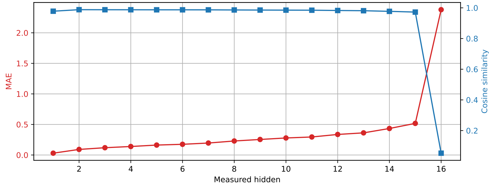
Llama-3.2-1B | Prompt 3 Spared layer 14 | Unquantized vs hybrid
