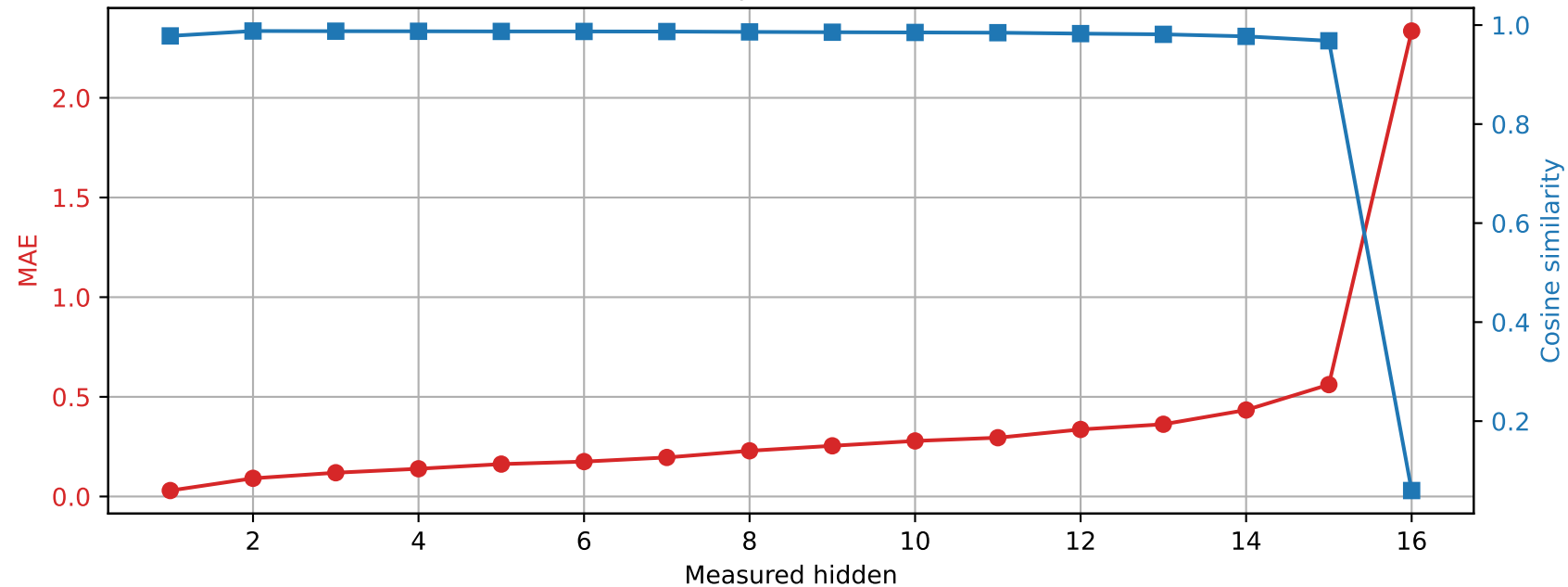
Llama-3.2-1B | Prompt 3 Spared layer 15 | Unquantized vs hybrid
