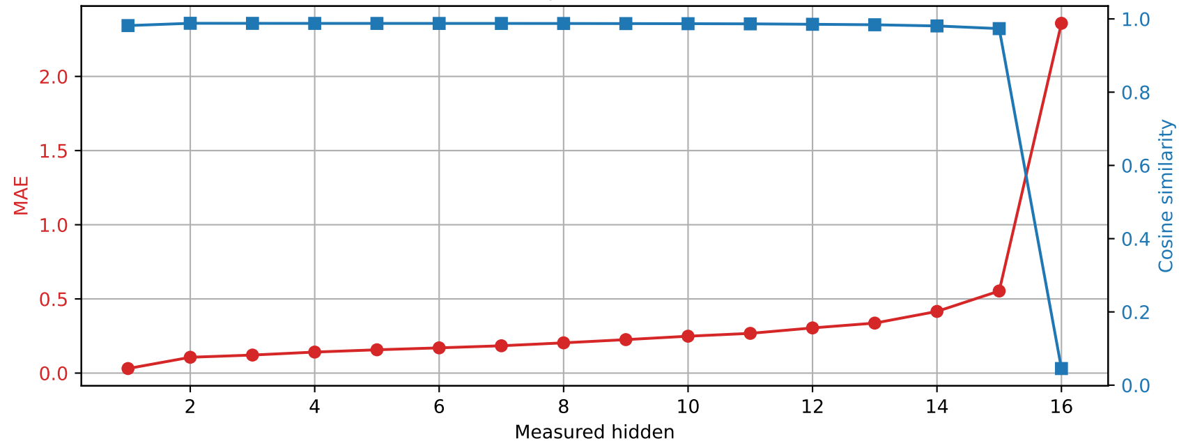
Llama-3.2-1B | Prompt 4 Spared layer 2 | Unquantized vs hybrid
