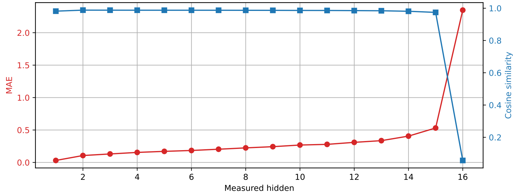
Llama-3.2-1B | Prompt 4 Spared layer 9 | Unquantized vs hybrid
