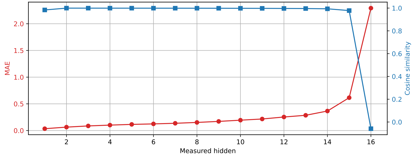
Llama-3.2-1B | Prompt 0 Spared layer 1 | Unquantized vs hybrid
