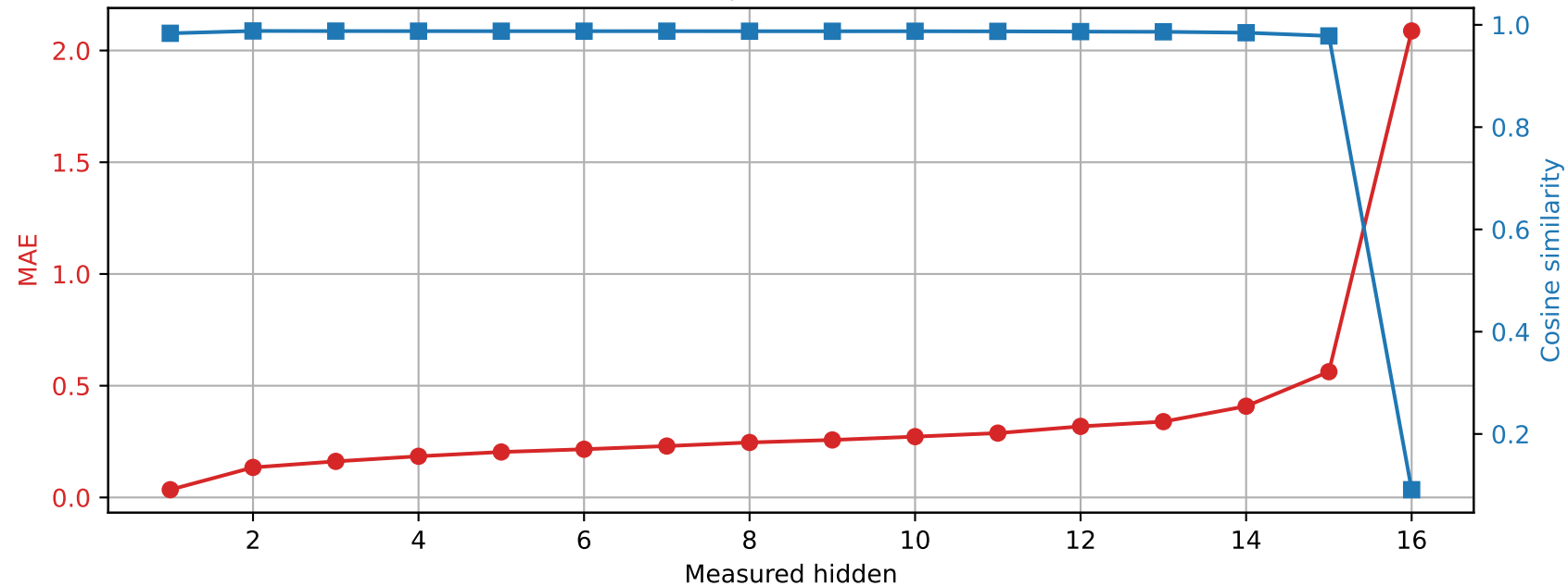
Llama-3.2-1B | Prompt 0 Spared layer 8 | Unquantized vs hybrid
