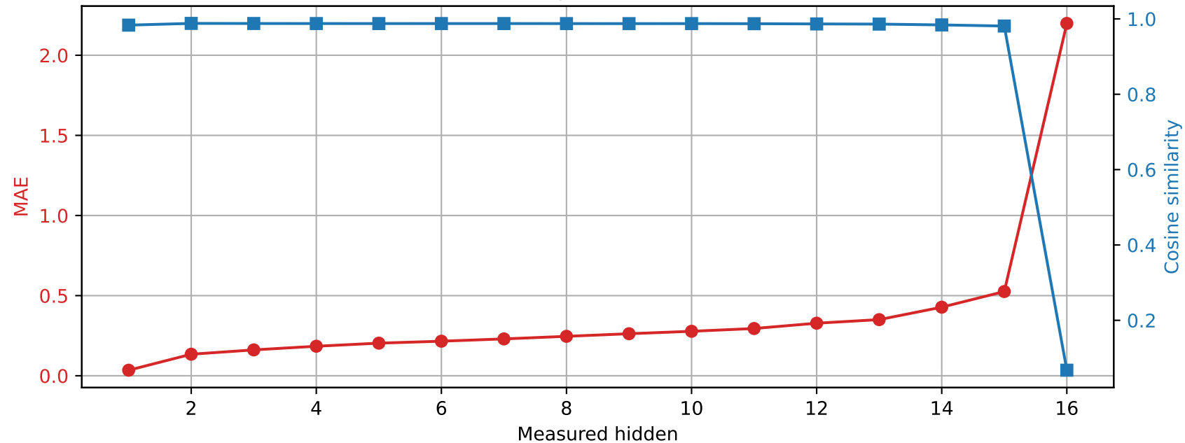
Llama-3.2-1B | Prompt 0 Spared layer 14 | Unquantized vs hybrid
