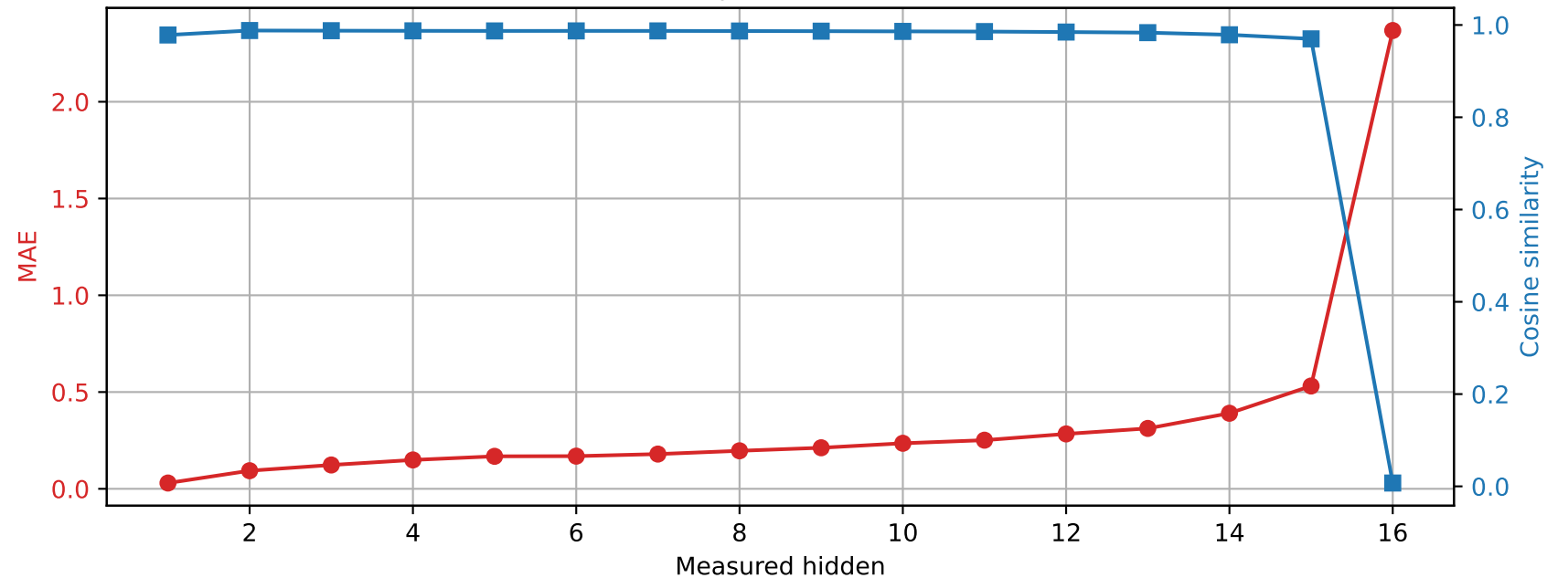
Llama-3.2-1B | Prompt 1 Spared layer 5 | Unquantized vs hybrid
