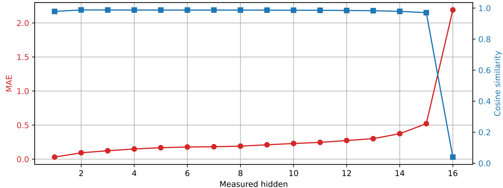
Llama-3.2-1B | Prompt 1 Spared layer 6 | Unquantized vs hybrid
