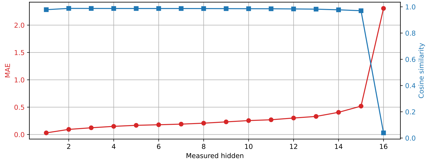
Llama-3.2-1B | Prompt 1 Spared layer 13 | Unquantized vs hybrid
