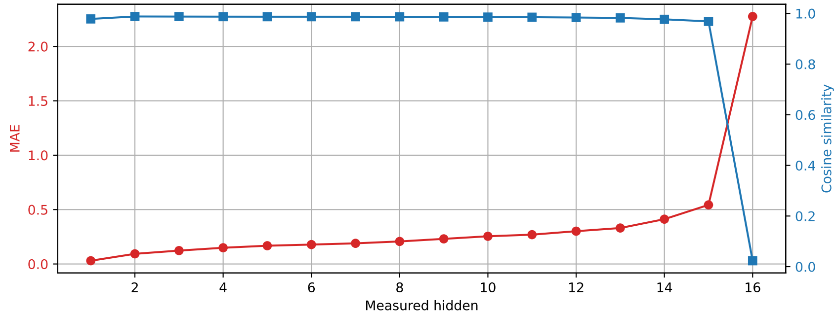
Llama-3.2-1B | Prompt 1 Spared layer 15 | Unquantized vs hybrid
