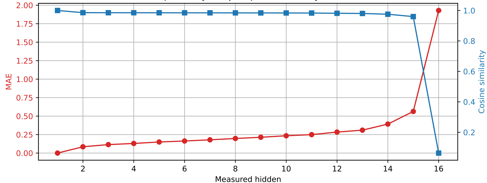
Llama-3.2-1B | Prompt 3 Spared layer 0 | Unquantized vs hybrid
