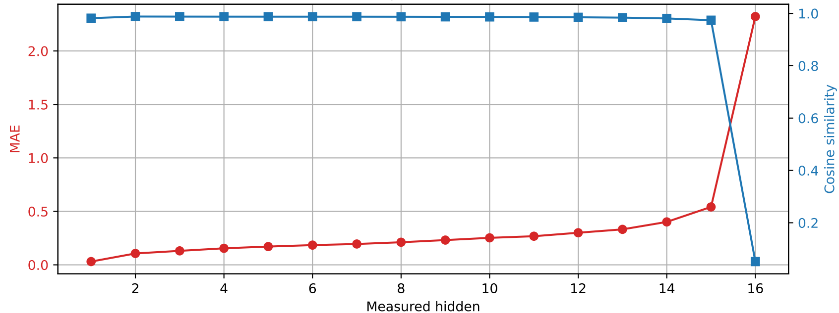
Llama-3.2-1B | Prompt 4 Spared layer 6 | Unquantized vs hybrid
