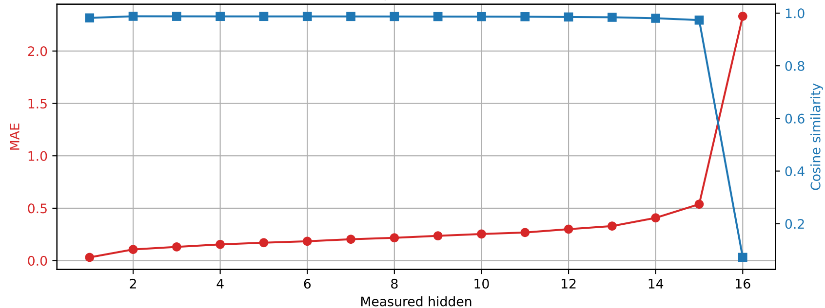
Llama-3.2-1B | Prompt 4 Spared layer 7 | Unquantized vs hybrid
