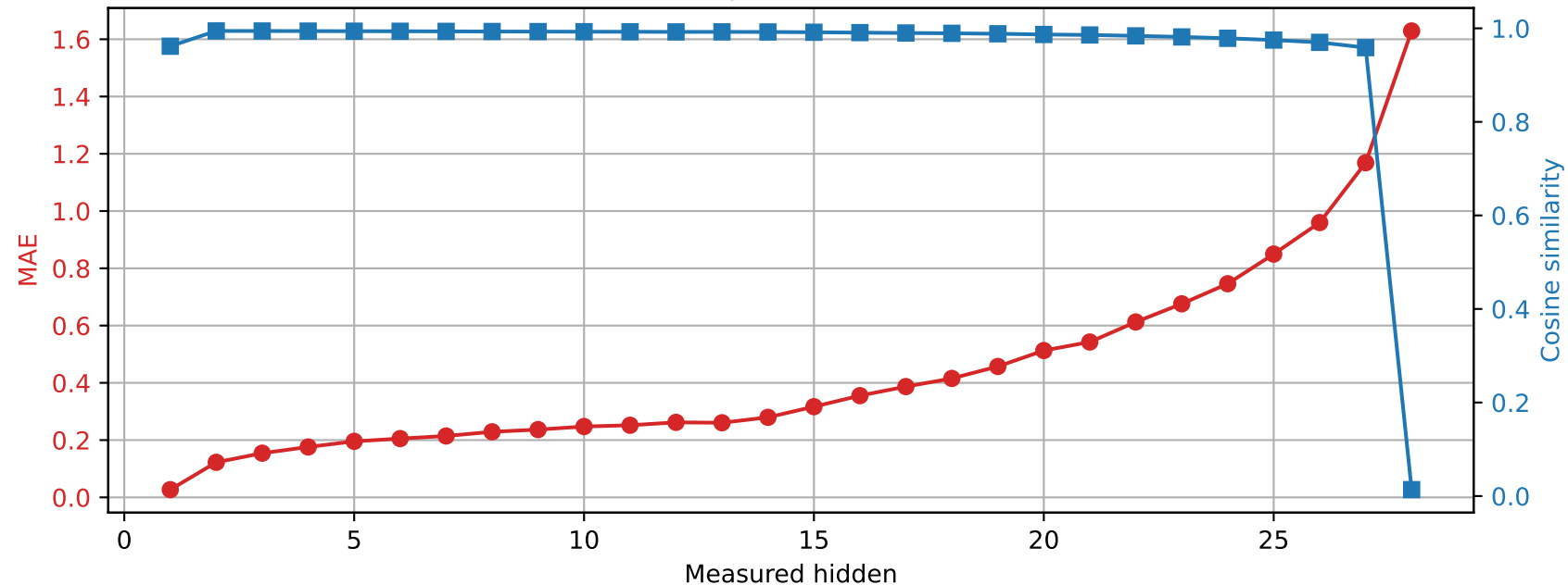
Llama-3.2-3B | Prompt 0 Spared layer 3 | Unquantized vs hybrid
