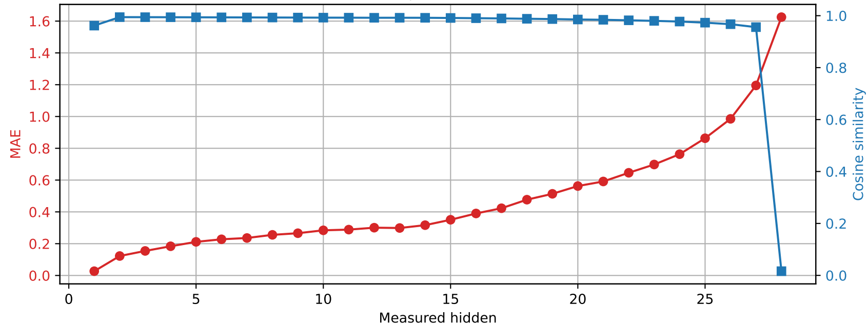
Llama-3.2-3B | Prompt 0 Spared layer 17 | Unquantized vs hybrid
