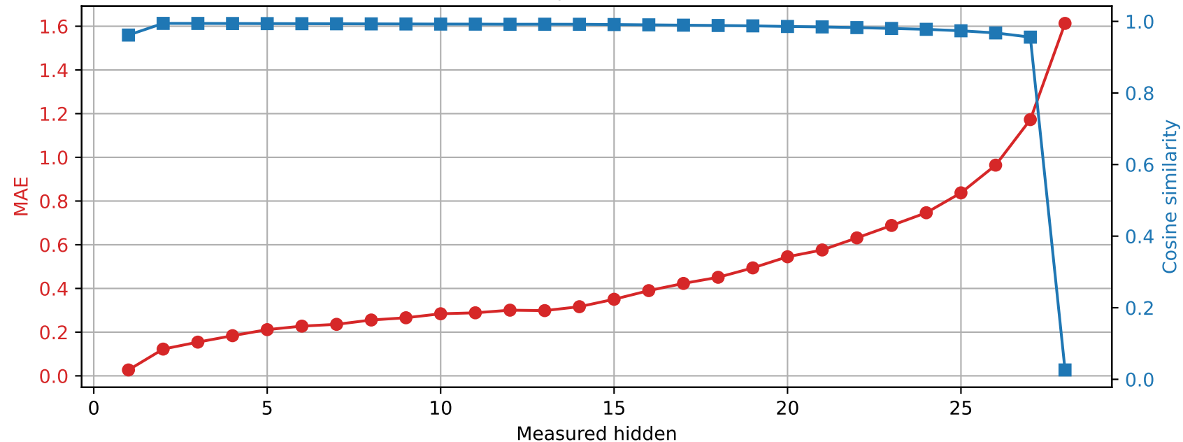
Llama-3.2-3B | Prompt 0 Spared layer 23 | Unquantized vs hybrid
