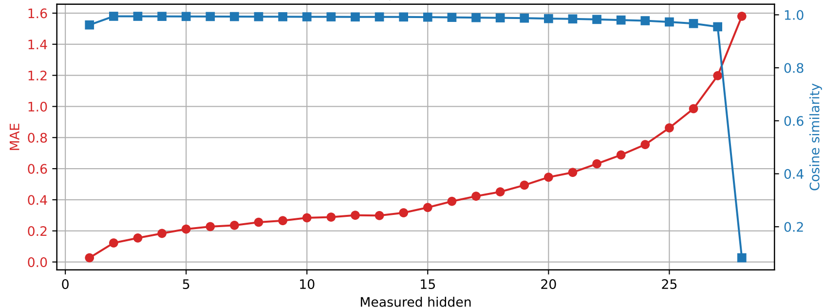
Llama-3.2-3B | Prompt 0 Spared layer 27 | Unquantized vs hybrid
