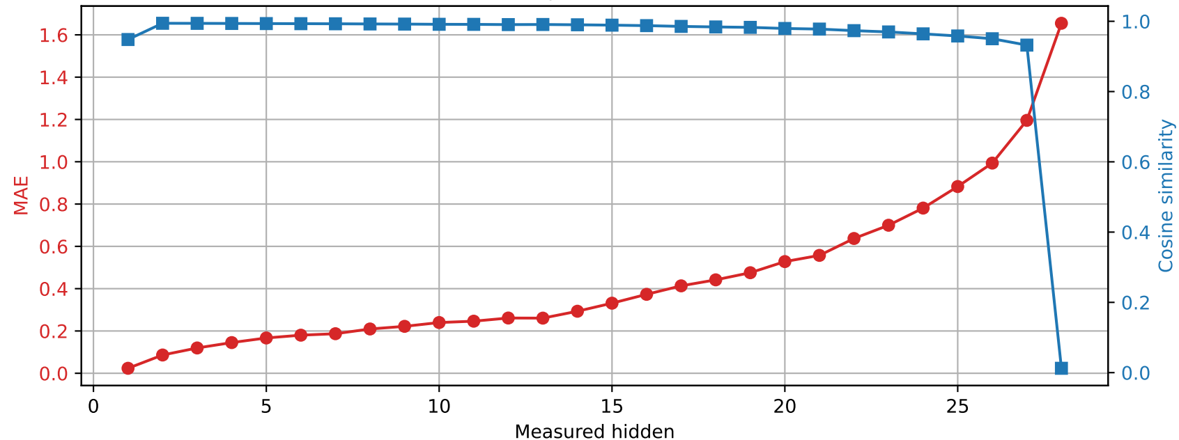
Llama-3.2-3B | Prompt 1 Spared layer 3 | Unquantized vs hybrid
