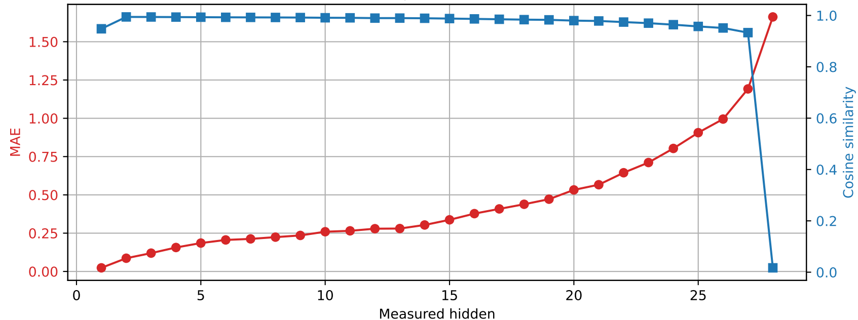
Llama-3.2-3B | Prompt 1 Spared layer 7 | Unquantized vs hybrid
