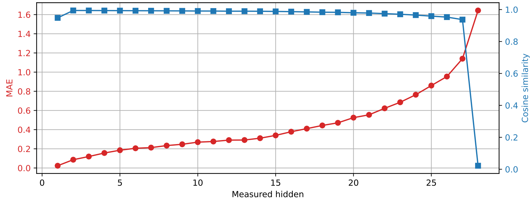
Llama-3.2-3B | Prompt 1 Spared layer 13 | Unquantized vs hybrid
