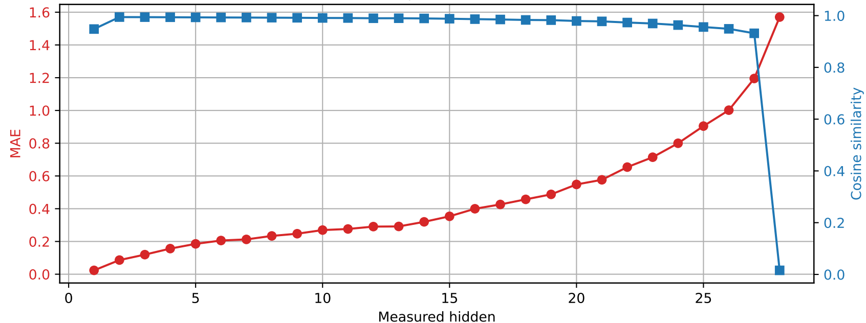
Llama-3.2-3B | Prompt 1 Spared layer 15 | Unquantized vs hybrid
