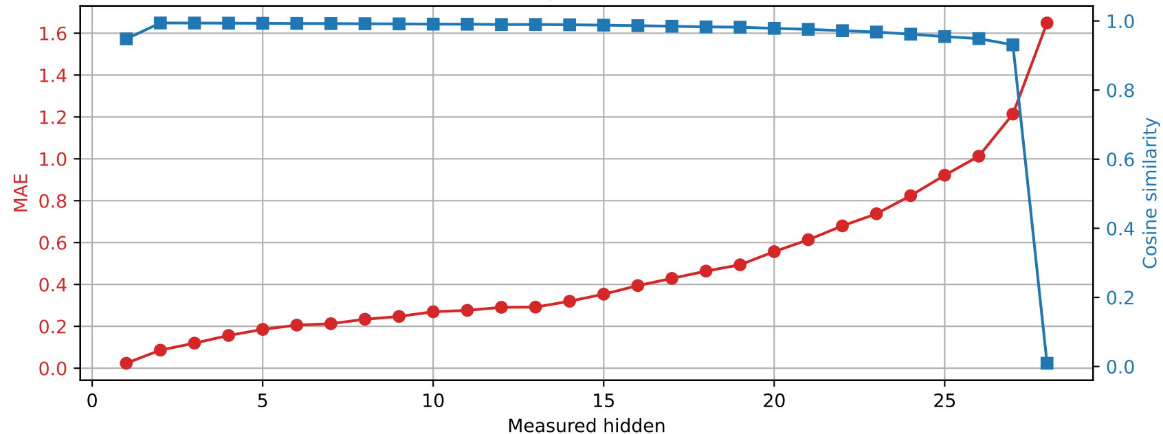
Llama-3.2-3B | Prompt 1 Spared layer 20 | Unquantized vs hybrid
