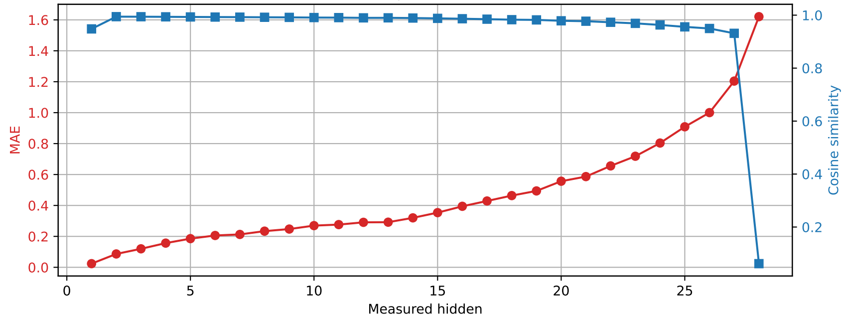
Llama-3.2-3B | Prompt 1 Spared layer 27 | Unquantized vs hybrid
