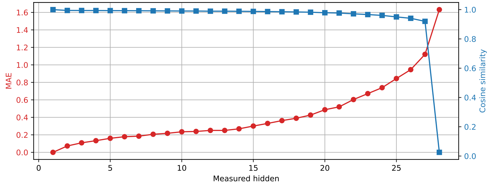
Llama-3.2-3B | Prompt 2 Spared layer 0 | Unquantized vs hybrid
