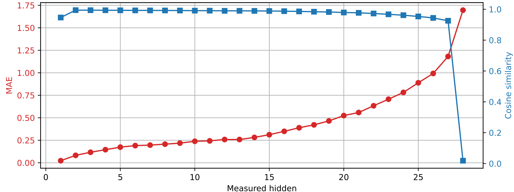
Llama-3.2-3B | Prompt 2 Spared layer 7 | Unquantized vs hybrid
