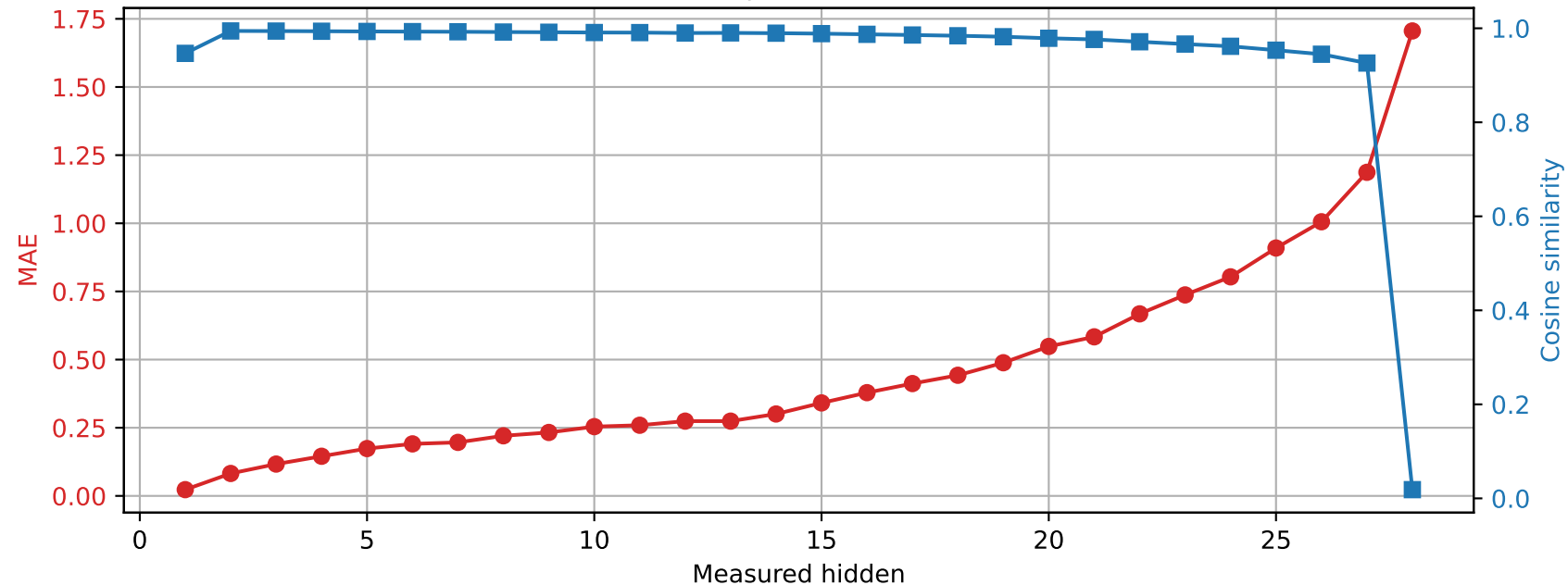
Llama-3.2-3B | Prompt 2 Spared layer 14 | Unquantized vs hybrid
