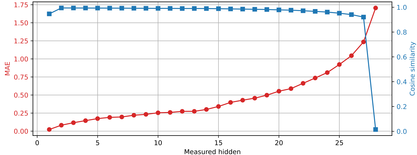
Llama-3.2-3B | Prompt 2 Spared layer 15 | Unquantized vs hybrid
