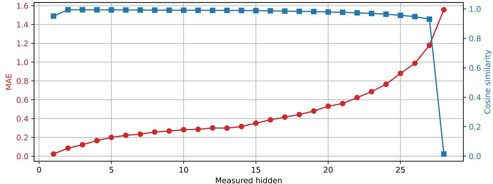
Llama-3.2-3B | Prompt 3 Spared layer 6 | Unquantized vs hybrid
