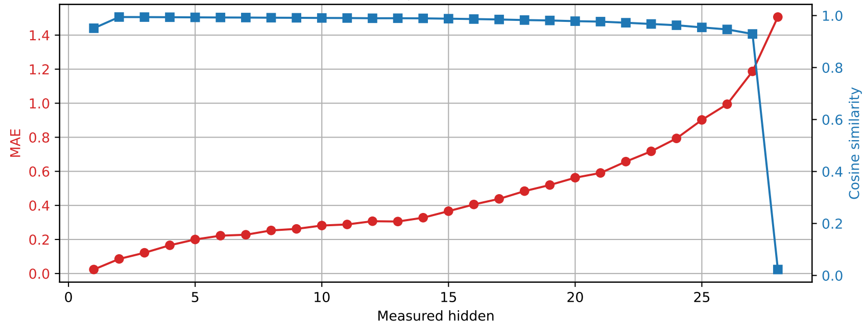
Llama-3.2-3B | Prompt 3 Spared layer 17 | Unquantized vs hybrid
