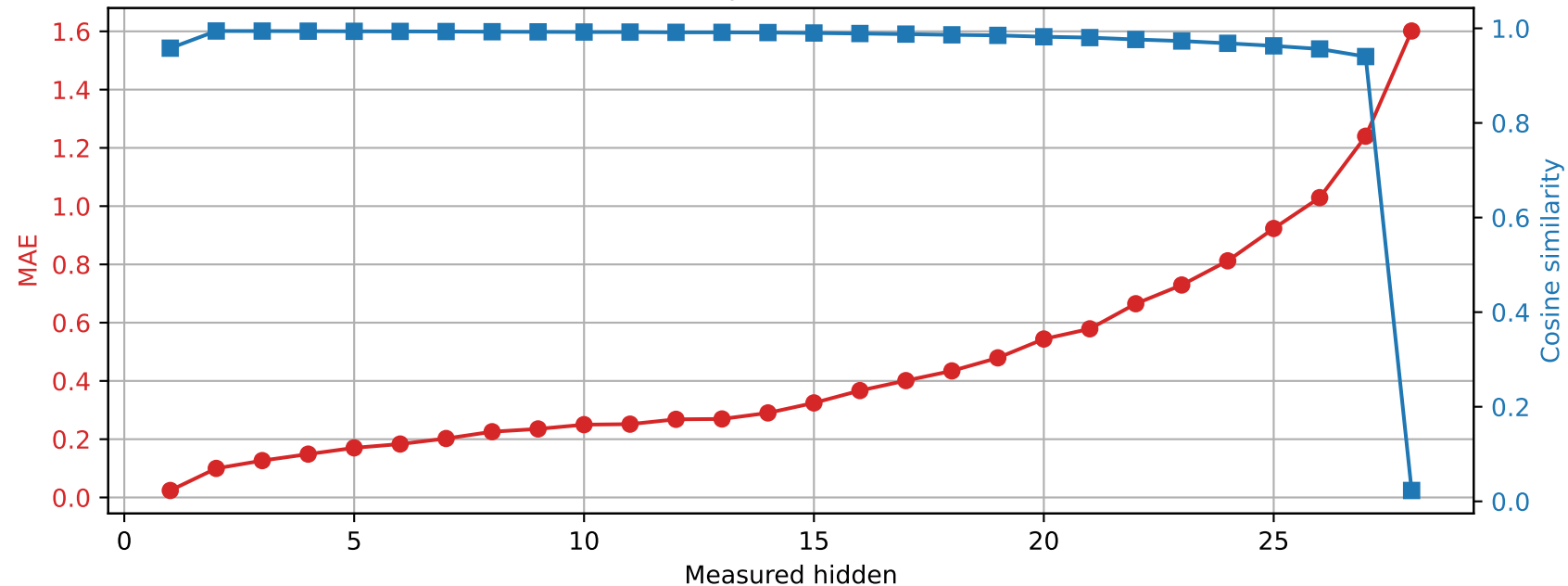
Llama-3.2-3B | Prompt 4 Spared layer 6 | Unquantized vs hybrid
