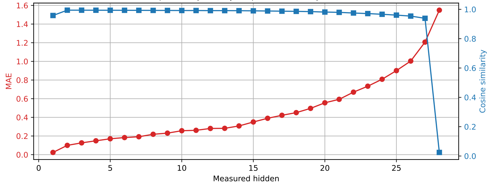
Llama-3.2-3B | Prompt 4 Spared layer 14 | Unquantized vs hybrid
