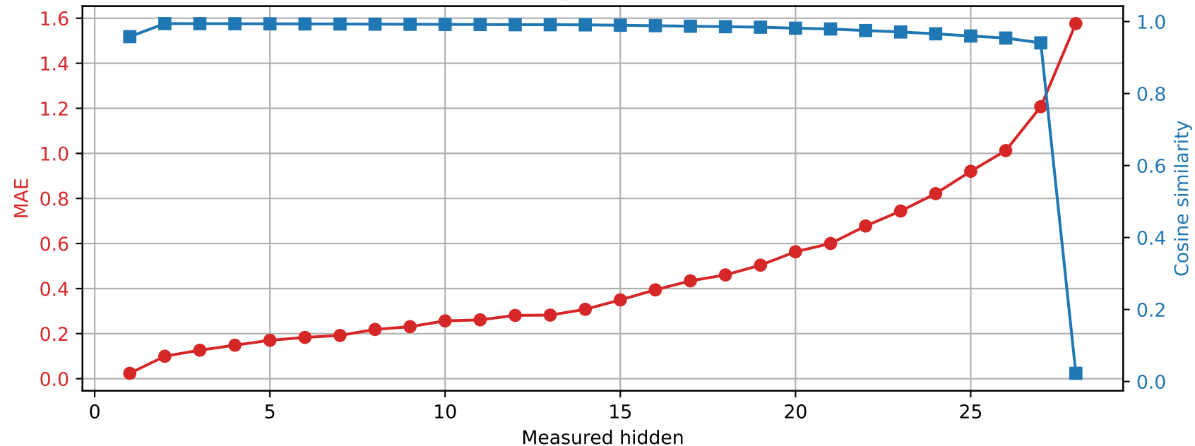
Llama-3.2-3B | Prompt 4 Spared layer 16 | Unquantized vs hybrid
