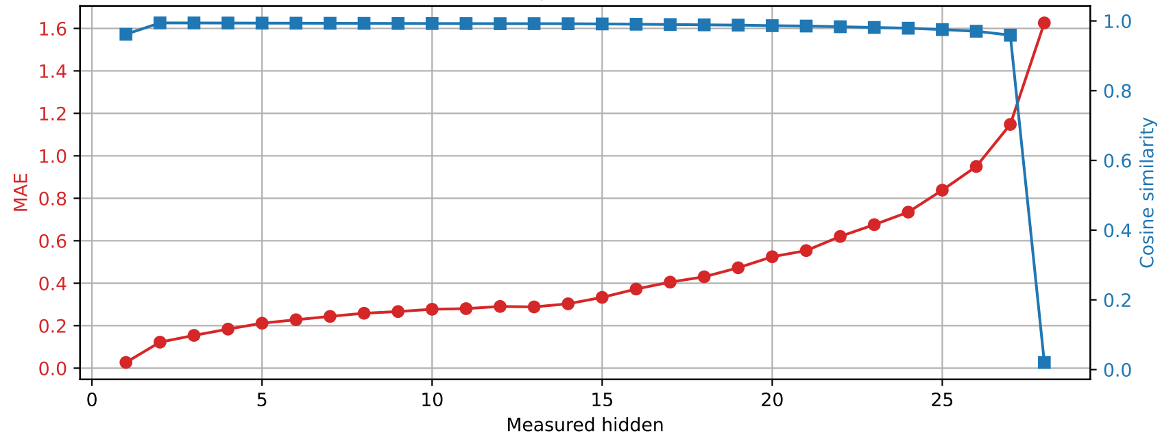
Llama-3.2-3B | Prompt 0 Spared layer 6 | Unquantized vs hybrid
