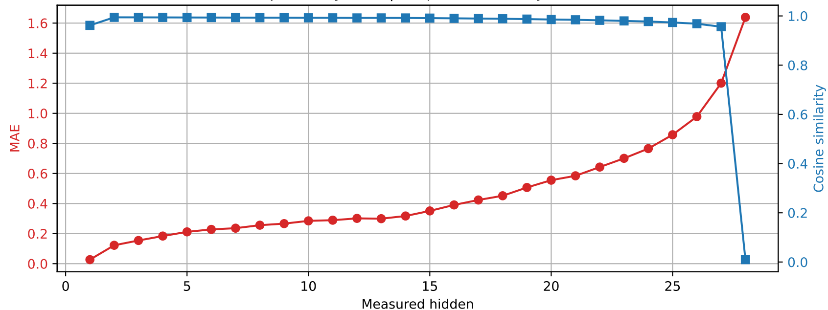
Llama-3.2-3B | Prompt 0 Spared layer 18 | Unquantized vs hybrid
