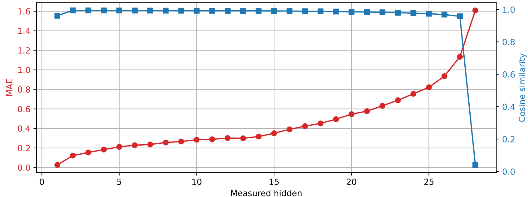
Llama-3.2-3B | Prompt 0 Spared layer 24 | Unquantized vs hybrid
