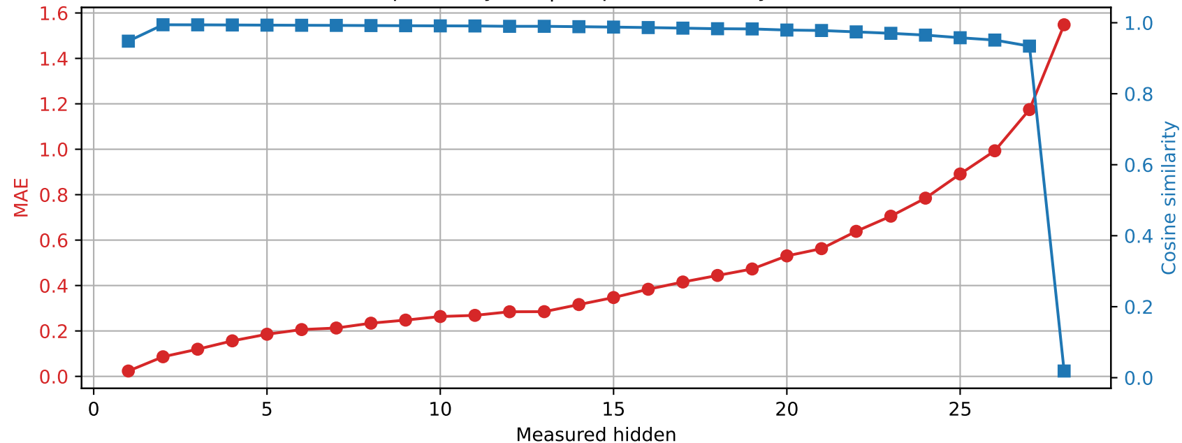
Llama-3.2-3B | Prompt 1 Spared layer 9 | Unquantized vs hybrid
