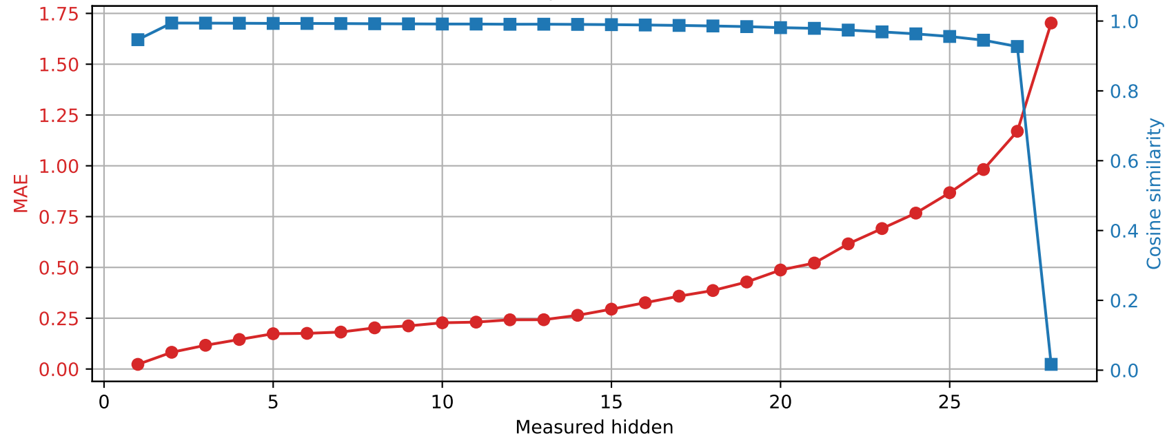
Llama-3.2-3B | Prompt 2 Spared layer 5 | Unquantized vs hybrid
