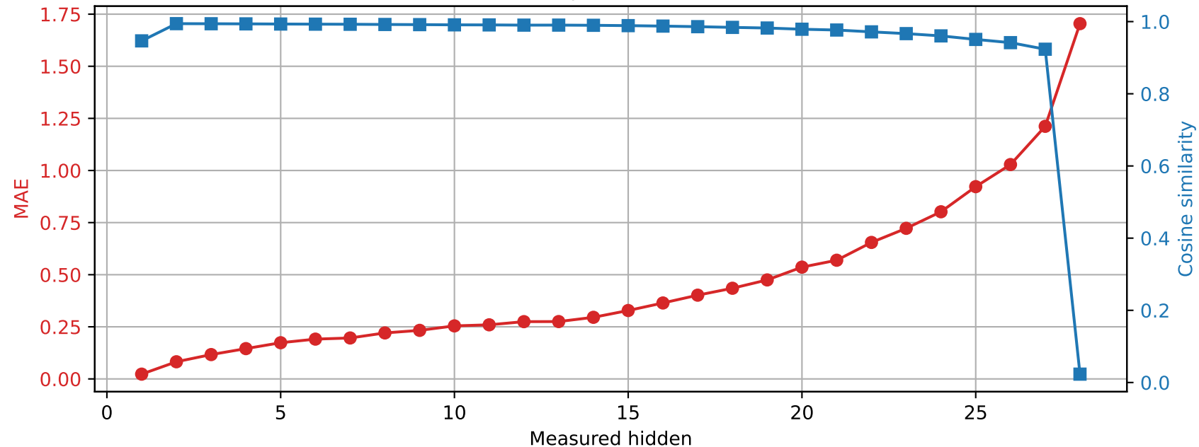
Llama-3.2-3B | Prompt 2 Spared layer 11 | Unquantized vs hybrid
